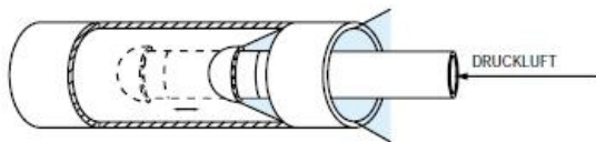
Schematische Zeichnung der Wirkungsweise von Rückblasdüsen in Rohren.
